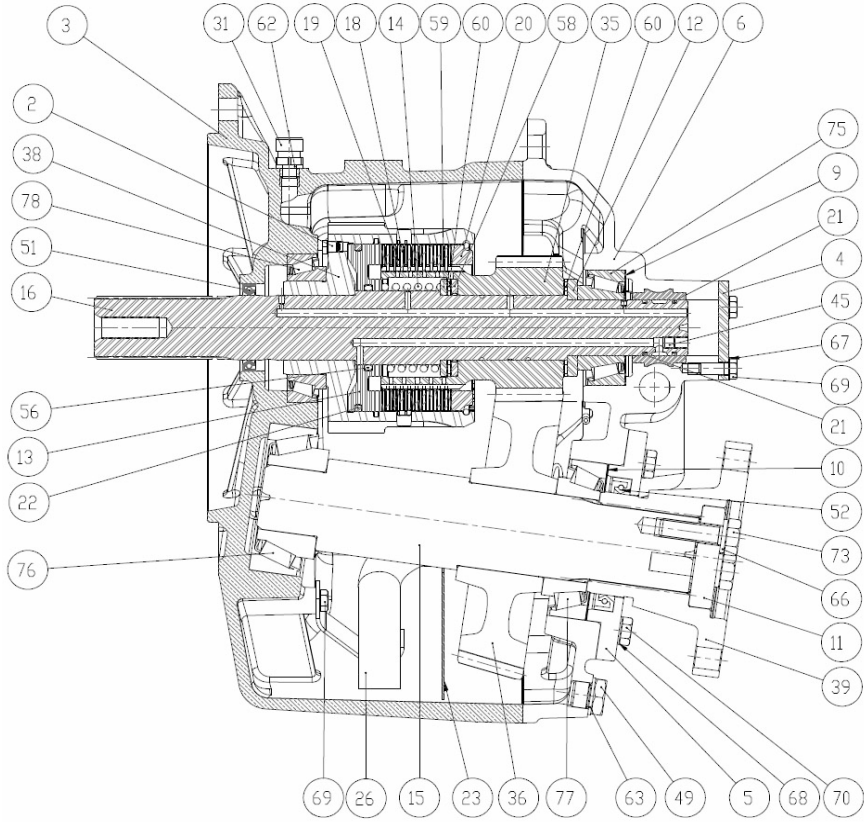
SEZIONE A-A
