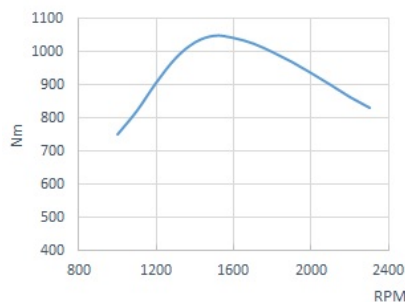
Vääntömomentti
