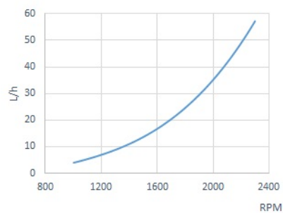
Polttoaineen kulutus
