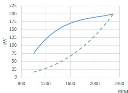
Teho ISO 3046/1 mukaan
